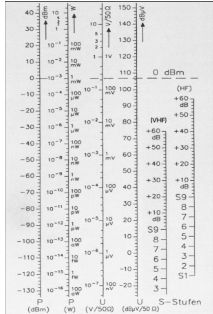
Beziehung zwischen S-Meteranzeige und Empfängereingangsspannung (nach DL2CH)
